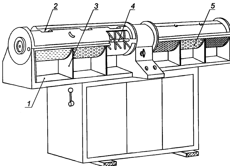
1 — рабочая камера; 2 — загрузочная воронка; 3 — перегородка; 4 — вал с колodkaми; 5 — сито
